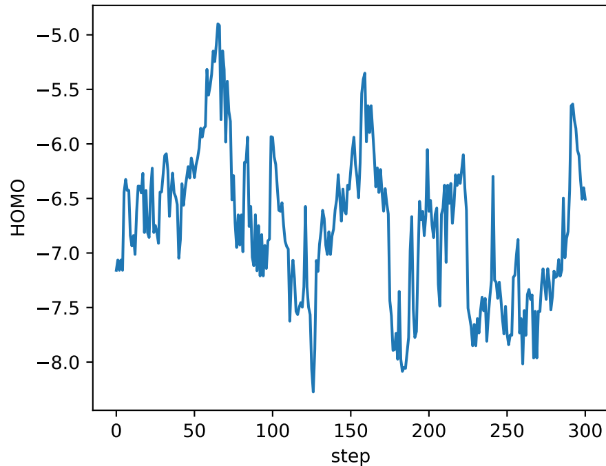
HOMO - evolution
