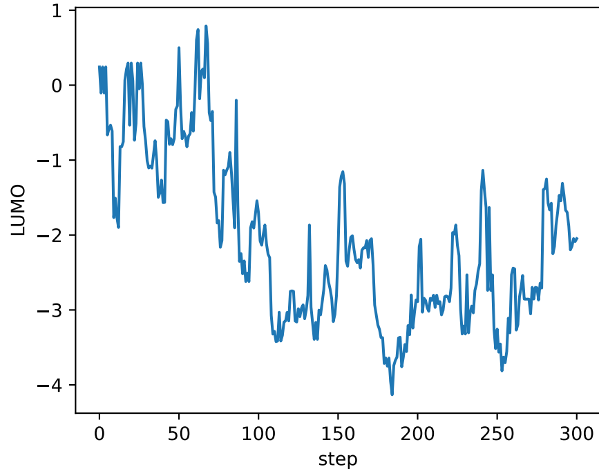
LUMO - evolution
